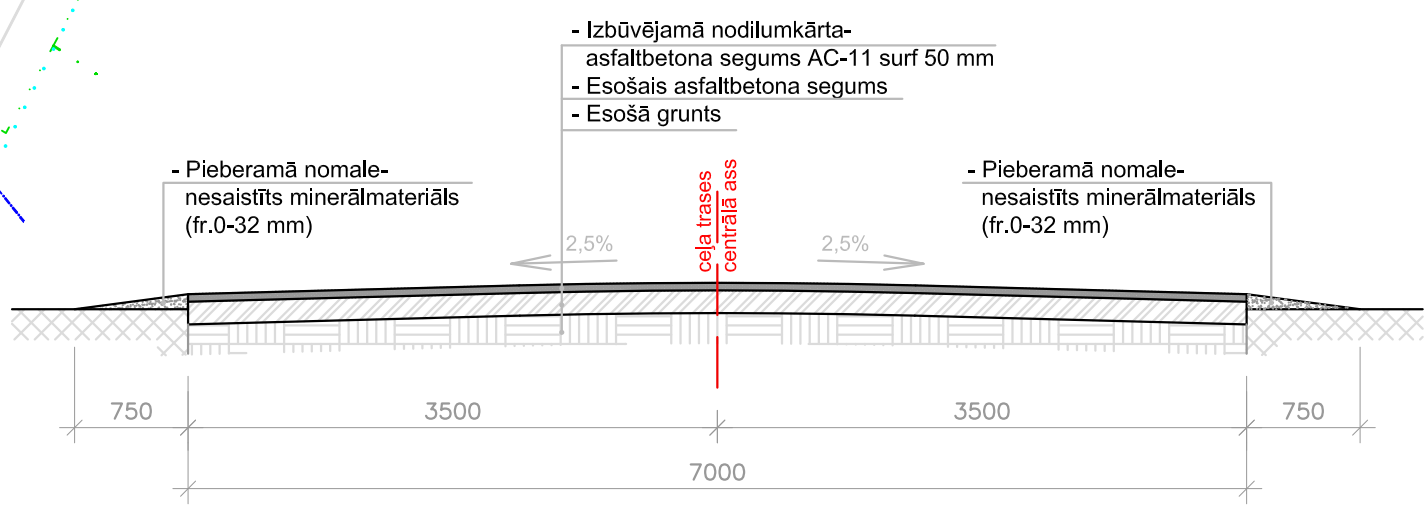
GRIEZUMS A - A M 1:50
