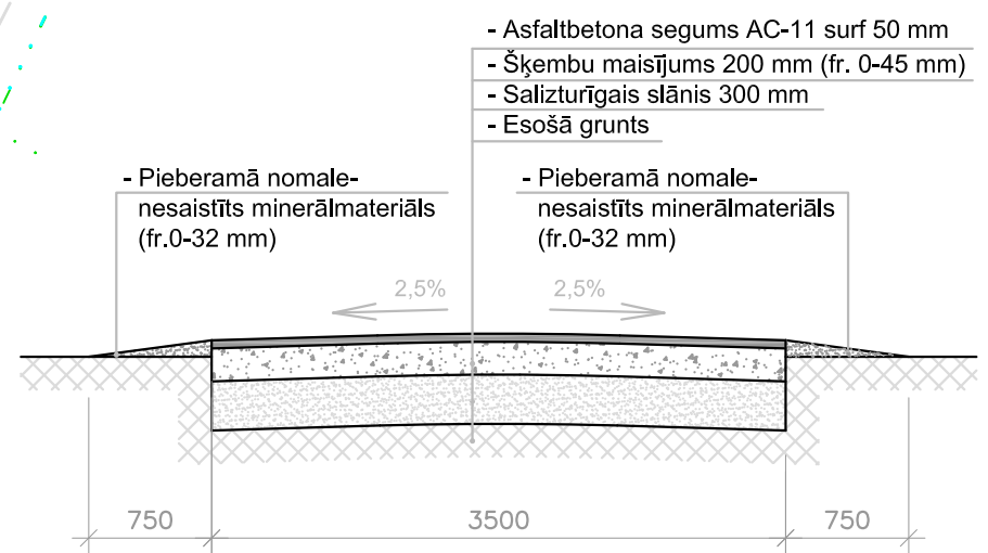
GRIEZUMS B - B M 1:50
